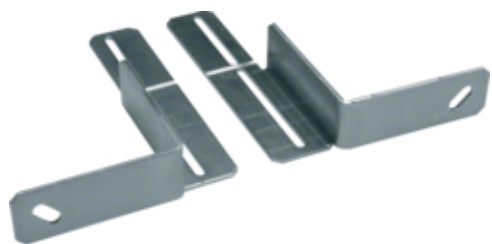
Inbouwset wandverdeler IP44/54
