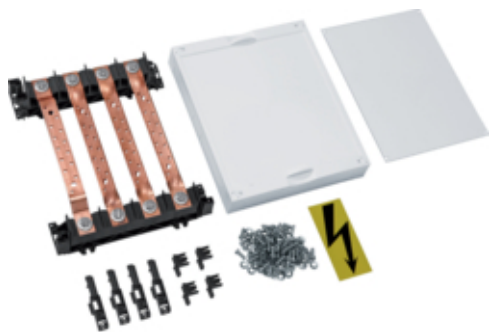
Verticale verdeelklem 4-polig 160 A, 25 x 4 mm
