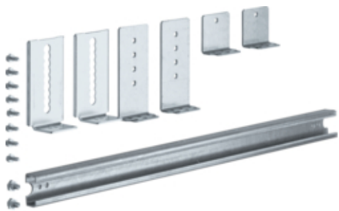
C-profiel met verdiepsbeugels, 2 velden 500 mm
