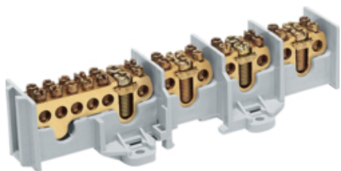
Verdeelklem 4-polig 1 x 35 mm 2 en 2/6 x 25 mm 2
