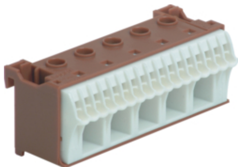
Aansluitklem fase, quickconnect, 22 posities
