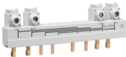
Doorverbindingsrail 20-40 A, 4-polig, voor HIM402/404
