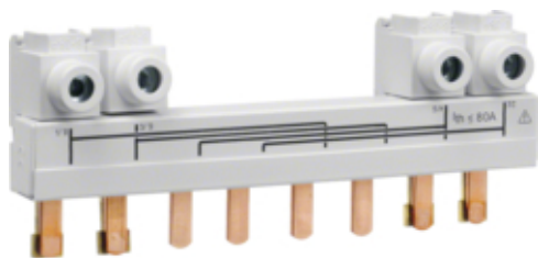
Doorverbindingsrail 63-80 A, 4-polig, voor HIM406/408
