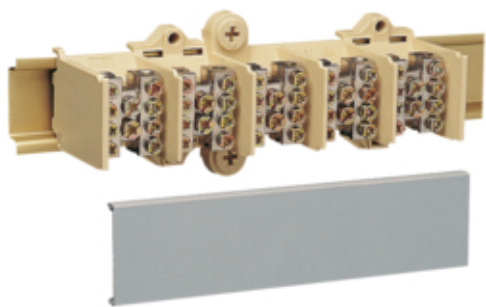
Verdeelklem 5-polig 1 x 25 mm 2 + 4 x 16 mm 2
